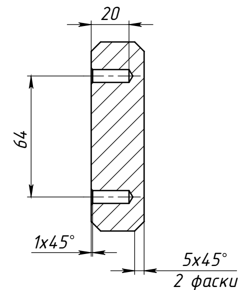
СЕЧЕНИЕ В-В МАСШТАБ 1 : 2
