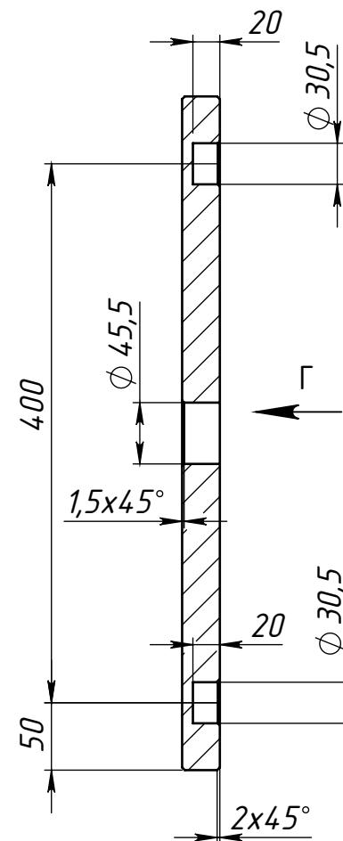
СЕЧЕНИЕ А-А
