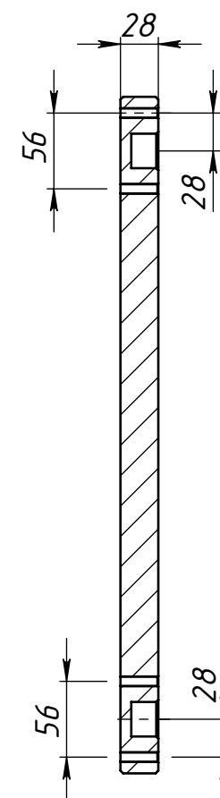
СЕЧЕНИЕ Б-Б
