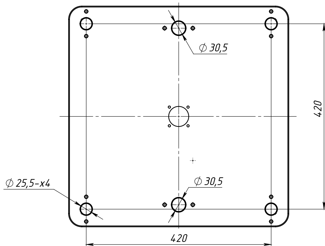
ВИД Г
